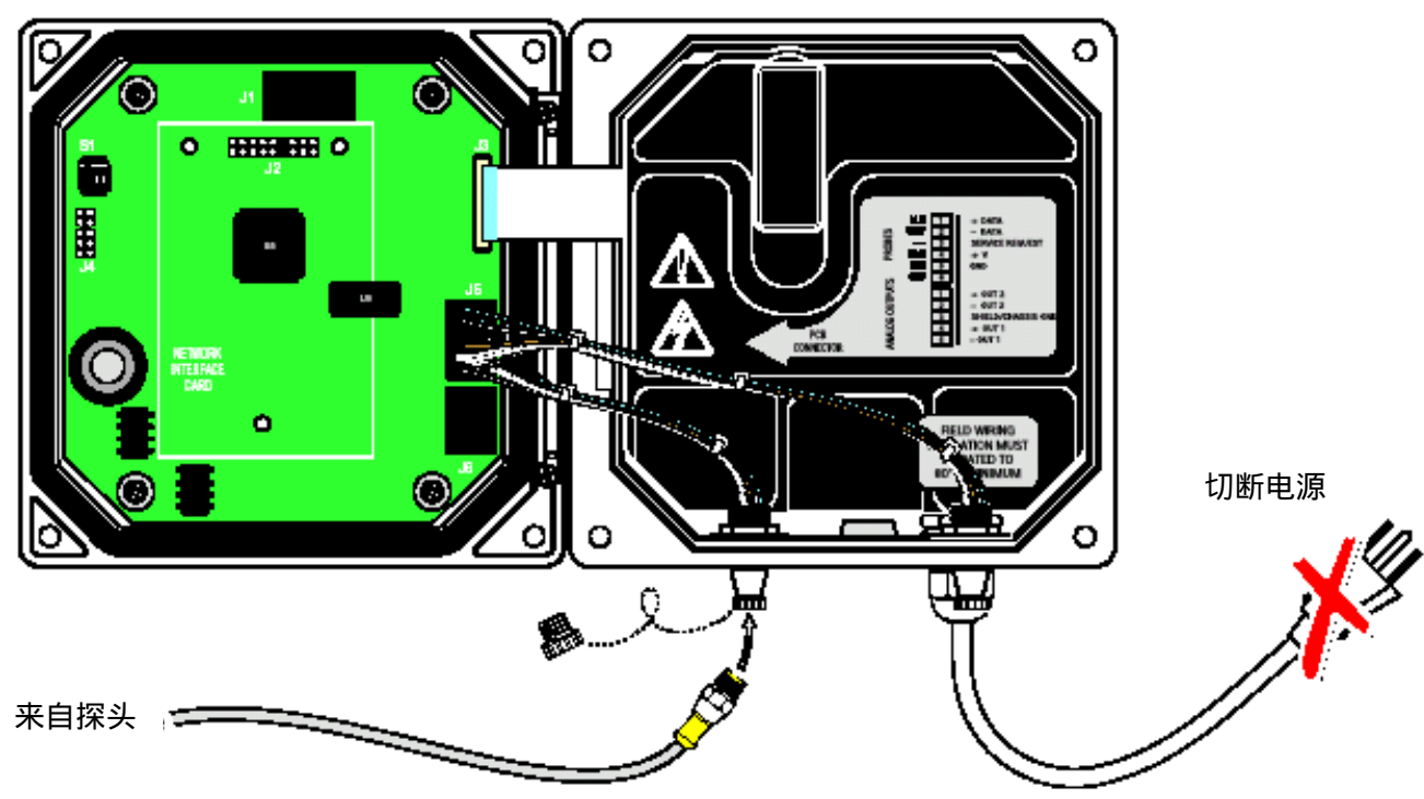
图 20 使用快速连接配件连接传感器
