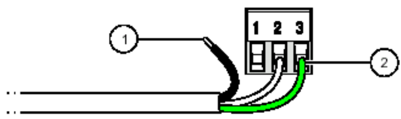
图 14 正确的导线准备及插入
